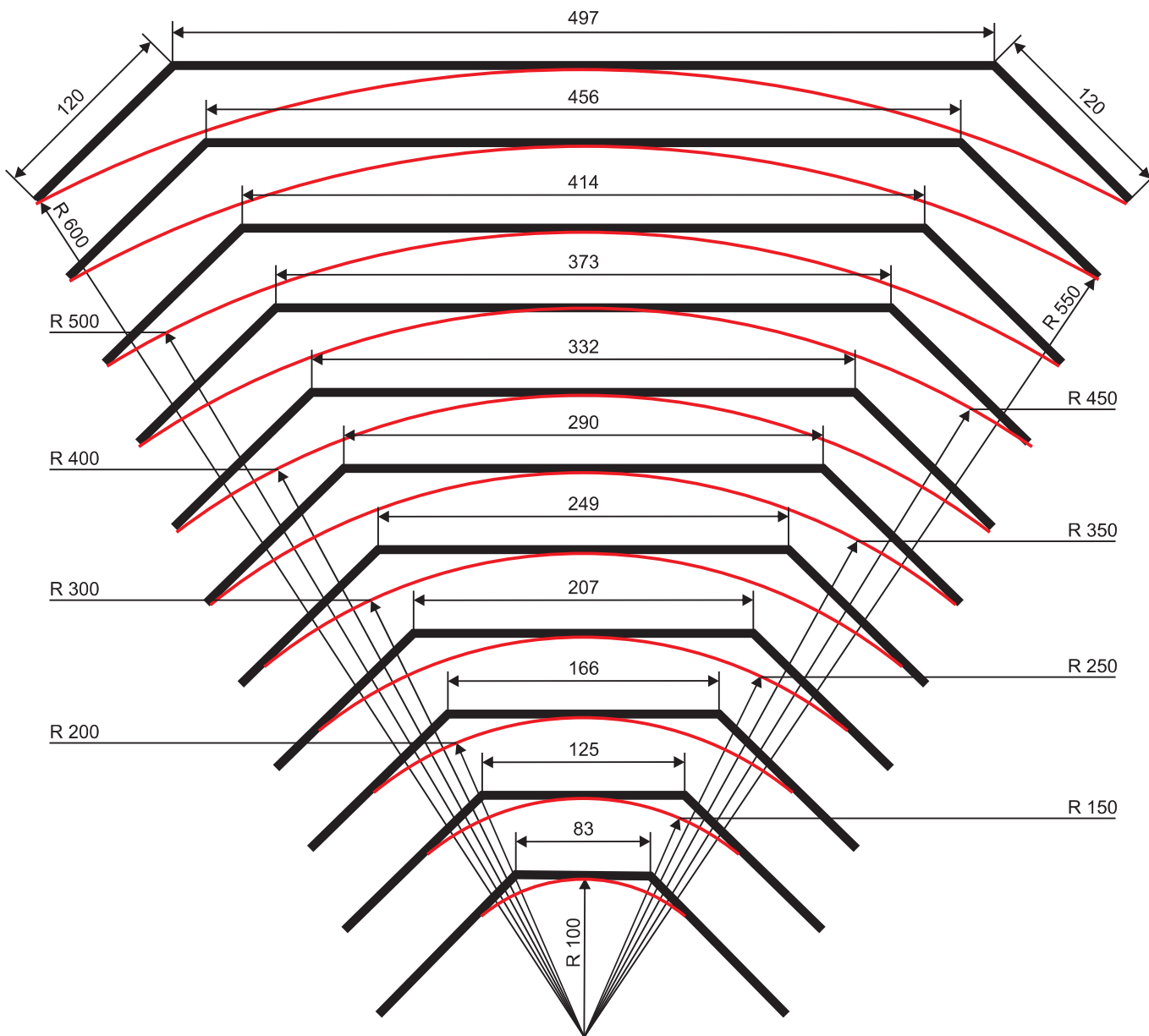
Radius Table
