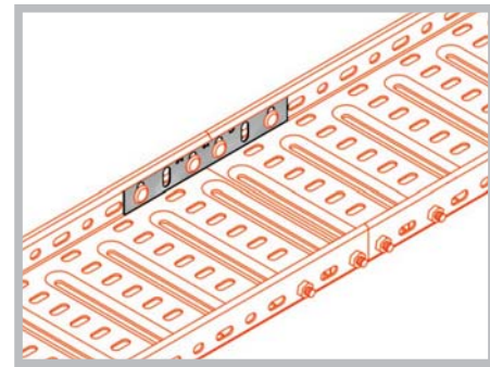
AN1-40-12 Connection Example
