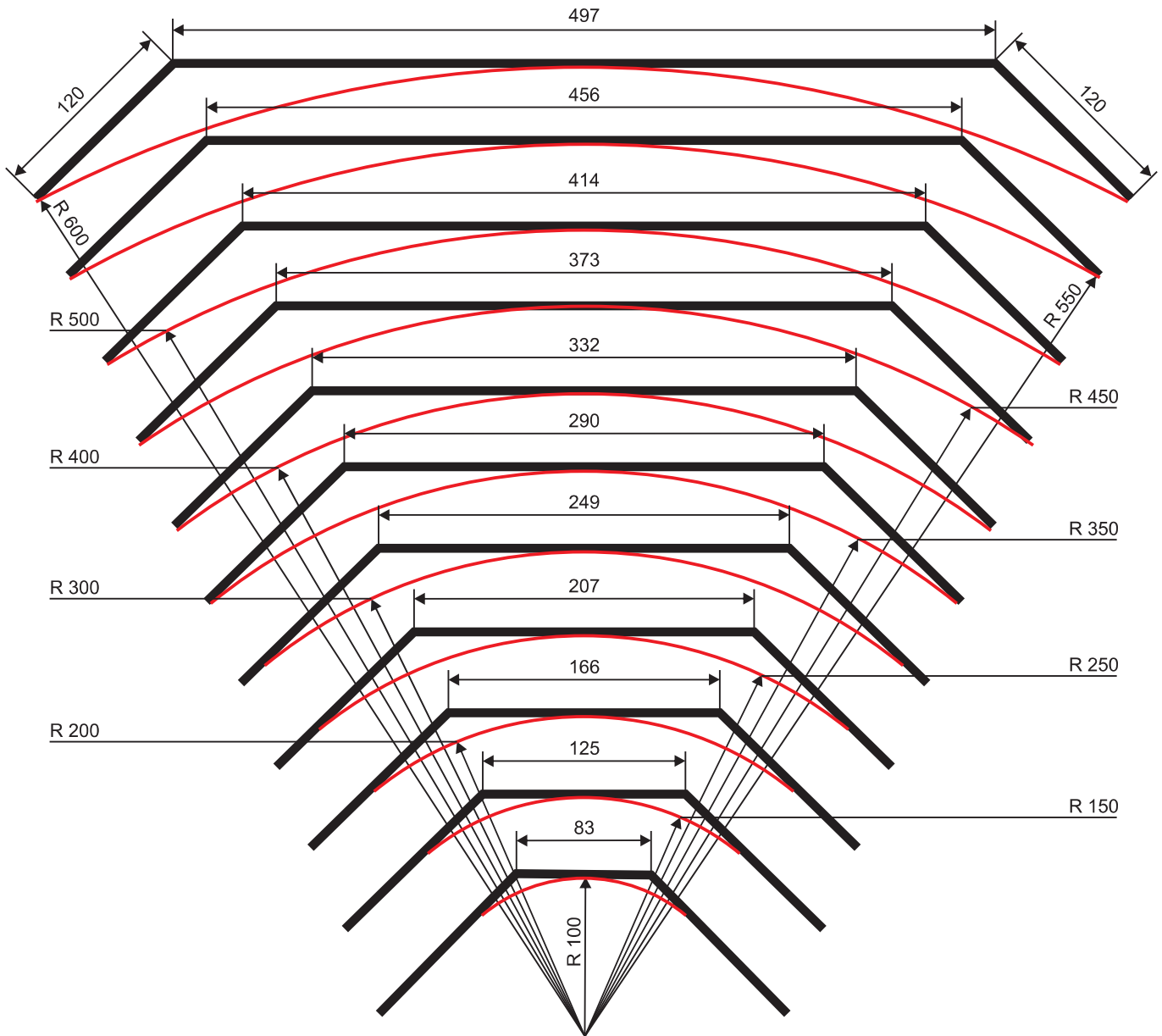
Radius Table
